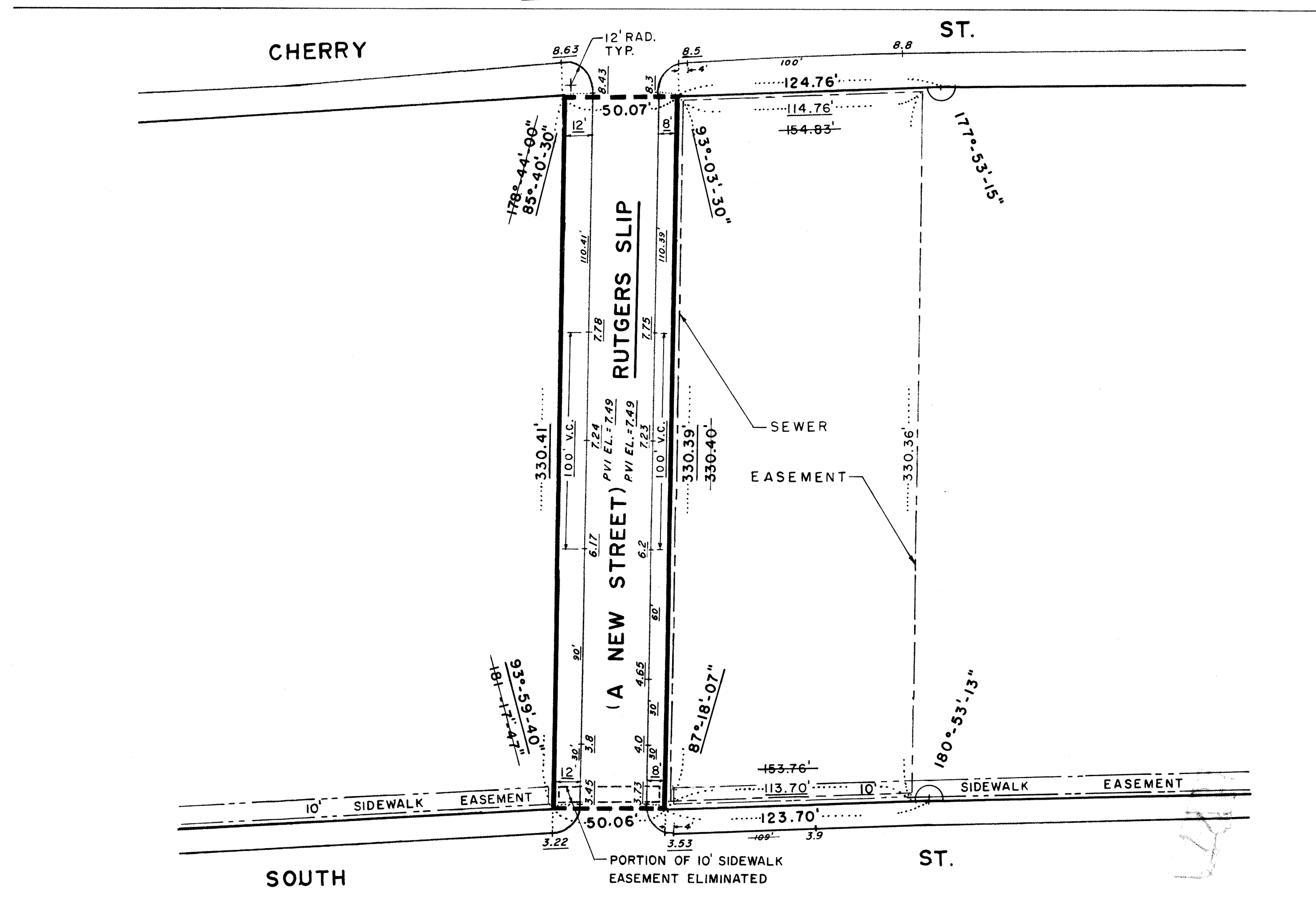
DETAIL "A" SCALE: 1" = 40'
