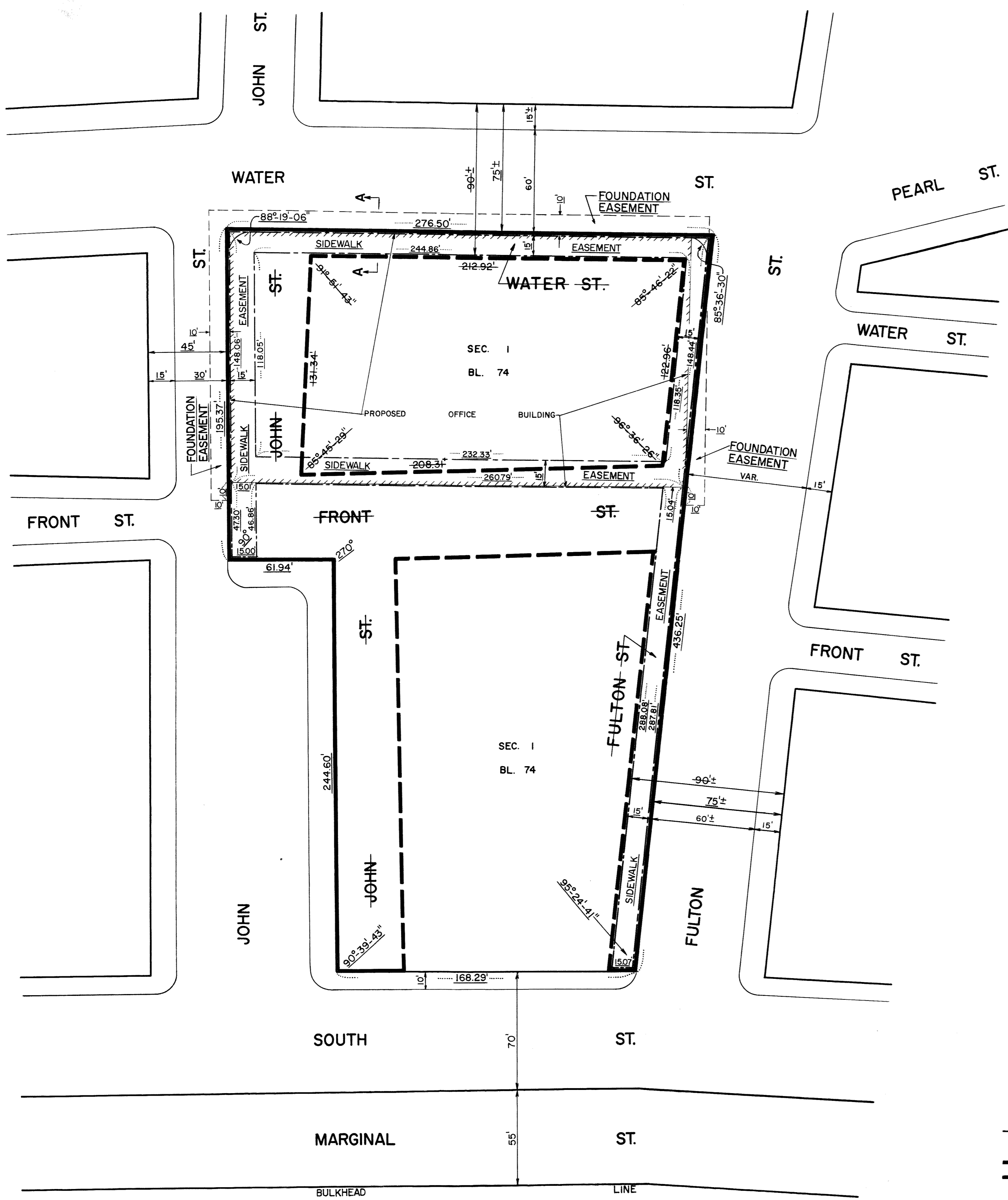
PLAN SCALE: 1"=40'
