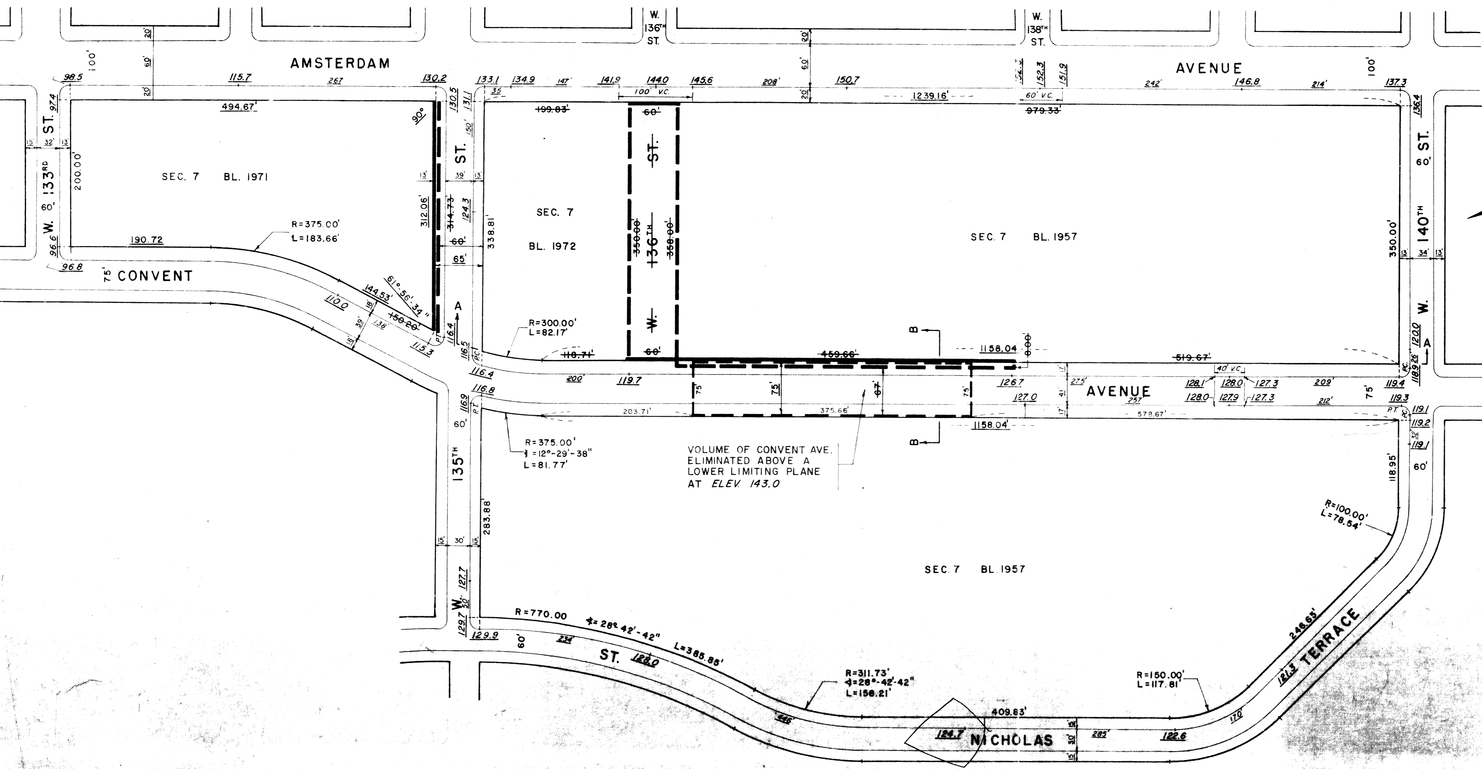
PLAN SCALE: 1"=80'
